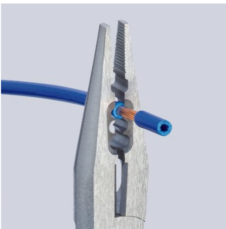
Dénudage 0,5 - 0,75 / 1,5 / 2,5 m²
