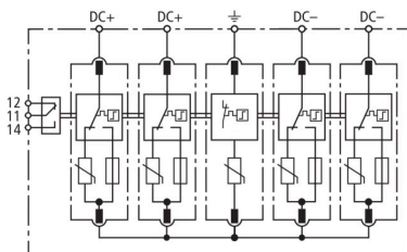
Schéma de principe du circuit DG M PV2 SCI 1000 FM
