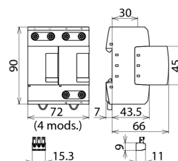
Dimensions DV M TT 2P 255 FM
