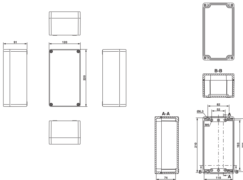
Dessin coté
