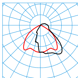
TX044680 DIN 5040: A40 UTE: 0,92 D + 0,08 T ■ C0 - C180 ■ C90 - C270
