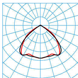
TX053203 UGR I = 19.4 UGR q = 18.2 DIN 5040: A40 UTE: 0,98 C + 0,02 T ■ C0 - C180 ■ C90 - C270
