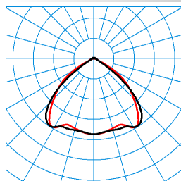
TX040384 UGR I = 20.9 UGR q = 19.9 DIN 5040: A40 UTE: 0,98 C + 0,02 T ■ C0 - C180 ■ C90 - C270
