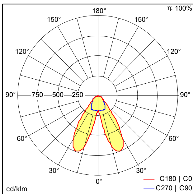
D43655AA_TECTON_C_LED7400-840_L2000_SB_LDE_SR.Idt
