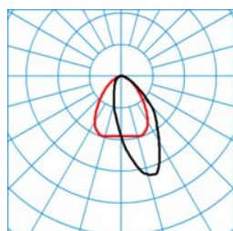
7850 HE LAN40-120 ML 830 L150 14 50 ■ C0 - C180
