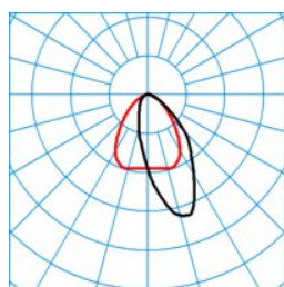
7850 HE LAN40-120 ML 830 L150 12 50 ■ C0 - C180
