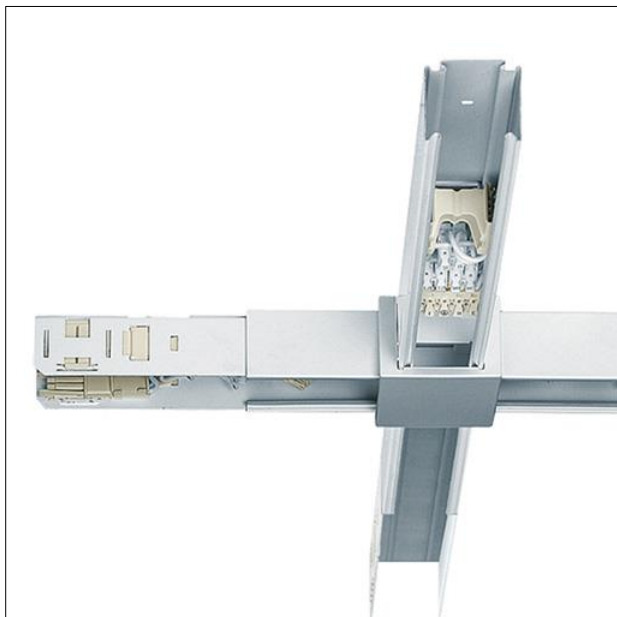
ZS_TEC_F_X-Knotenverbinder.jpg
