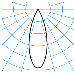
7651 LentyP L-FL 40-835 M34 ETBLE 01 (225) TX775973 ■ C0 - C180 ■ C90 - C270
