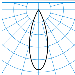
7651 LentyP L-FL 40-835 M34 ETBLE 01 (150) TX775972 ■ C0 - C180 ■ C90 - C270
