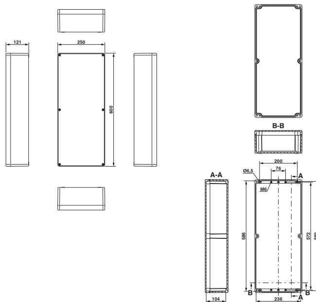
Dessin coté
