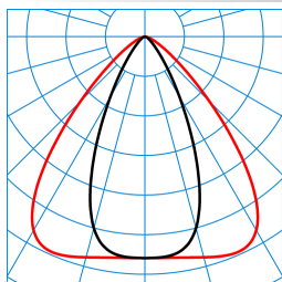
Grado 3P WRS-DF84-o 40-835 M42 ET 03 TX570438
