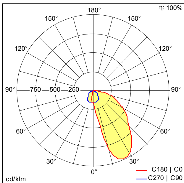
D34983AA_TECTON_C_LED7400-865_L2000_WW_LDE_SR.Idt
