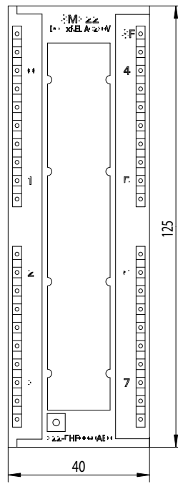
Vorne / Front
