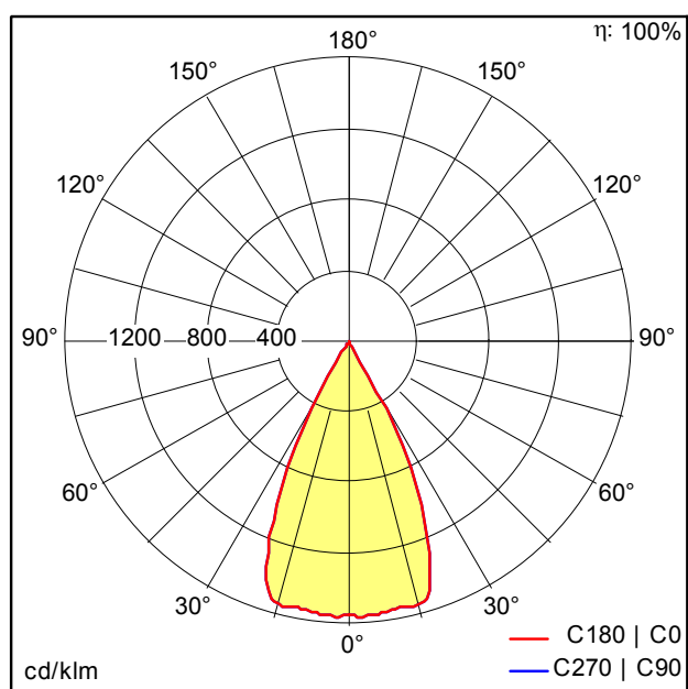
STx585.idt
