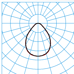
ArimoFit M48 PW19 53-840 TX369908 ■ C0 - C180 ■ C90 - C270 UGR I = 18,4 UGR q = 18,3 DIN 5040: A50 UTE: 1,00 C CEN Flux Code: 65 89 97 100 100 0 0 0 0
