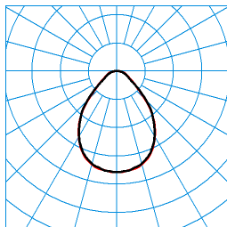
ArimoFit M48 PW19 53-840 ET TX429026 ■ C0 - C180 ■ C90 - C270 UGR I = 18,4 UGR q = 18,3 DIN 5040: A50 UTE: 1,00 C CEN Flux Code: 65 89 97 100 100 0 0 0 0
