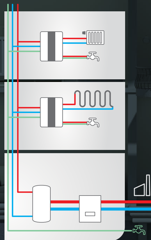
Systeme moderne à 3 colonnes avec distribution de chauffage et production d'ECS décentralisée
