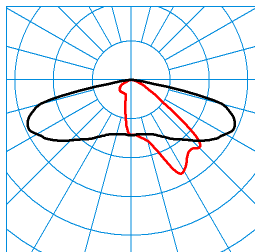
Jovie 50-AB2L-ML/1000-2200-740 2G1 ETDD (1500 lm) TX068679 ■ C0 - C180 ■ C90 - C270 DIN 5040: A30 UTE: 0,98 l CEN Flux Code: 34 70 96 100 98
