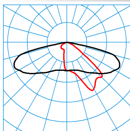
Jovie 50-AB2L-ML/1000-2200-740 2G1 ETDD (1000 lm) TX068678 ■ C0 - C180 ■ C90 - C270 DIN 5040: A30 UTE: 0,98 l CEN Flux Code: 34 70 96 100 98
