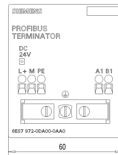
Vorne / Front
