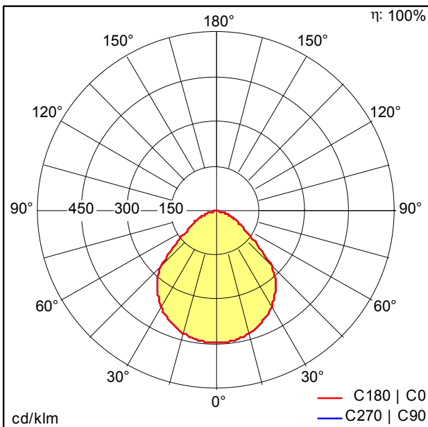
D37139AA_u_ONDA2_E_LRO_D590_LED3400-927-65.idt
