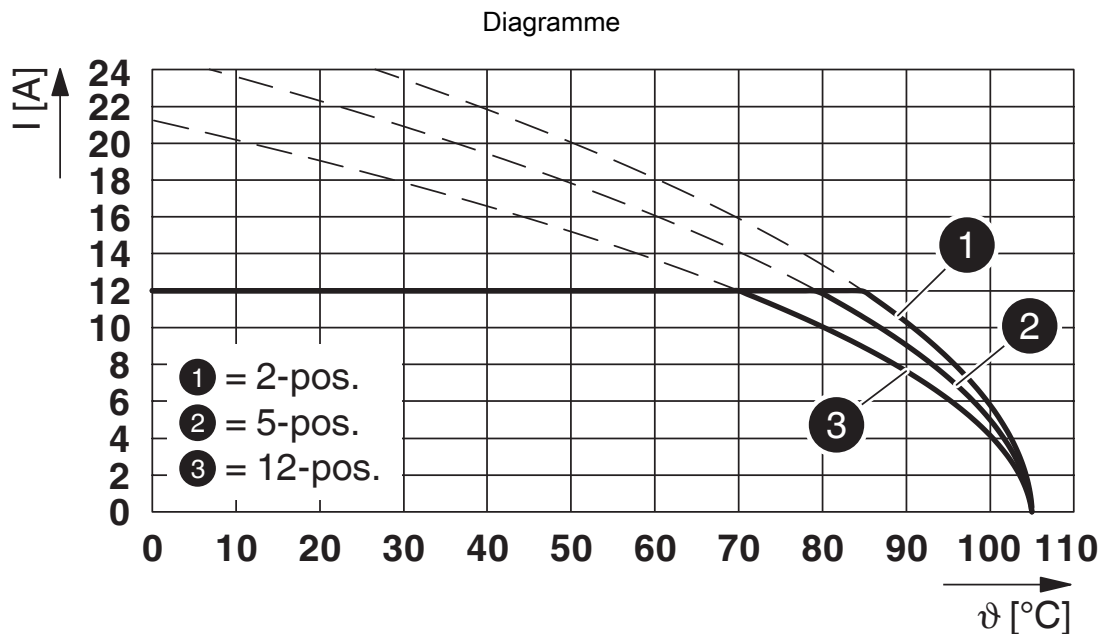
Type : FKCS 2,5/...-STF-5,08 avec CCV 2,5/...-GF-5,08-LR P...THR
