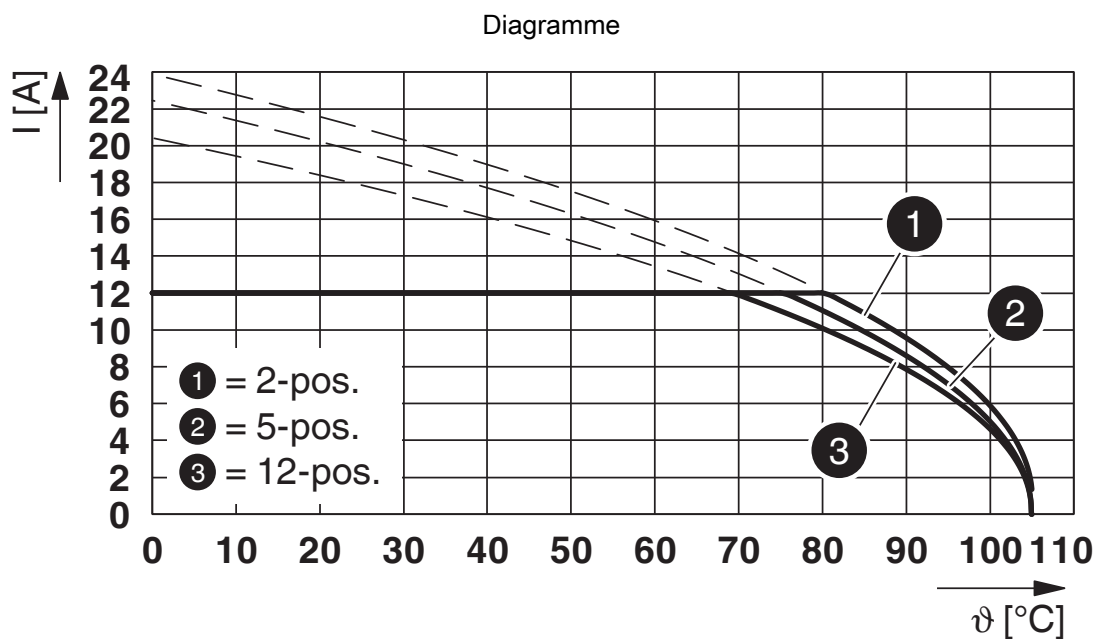
Type : FKCS 2,5/...-STF-5,08 avec CCV 2,5/...-GF-5,08 P...THR
