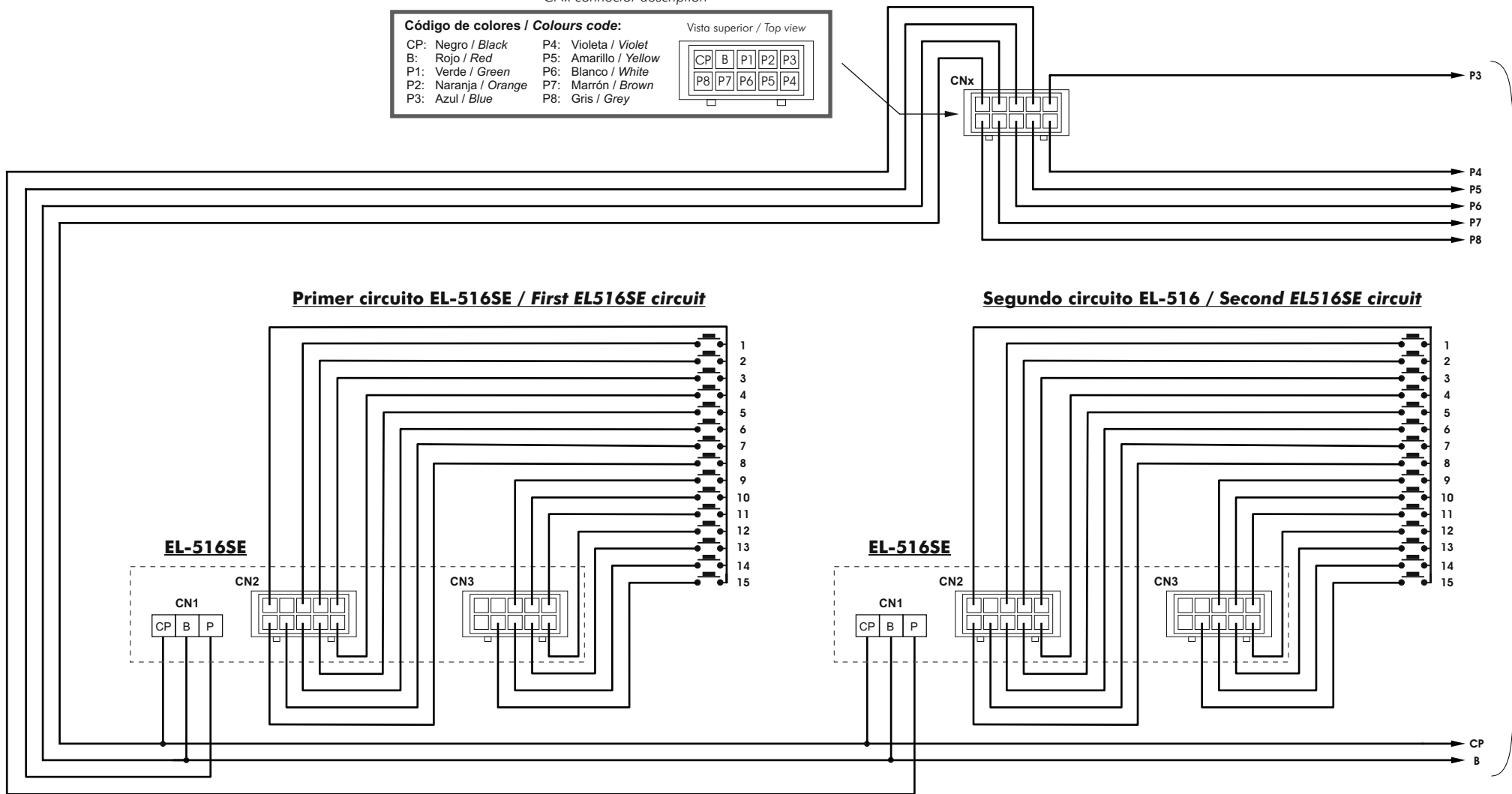
EL516SE Descripción conector CN2 / CN2 connector description
