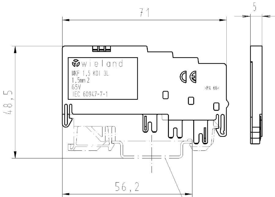
Hutschiene EN 60715-35x7,5 mounting rail EN 60715-35x7,5
