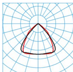
7850 LW2255-140 ML 830 L225 14 50 ■ C0 - C180
