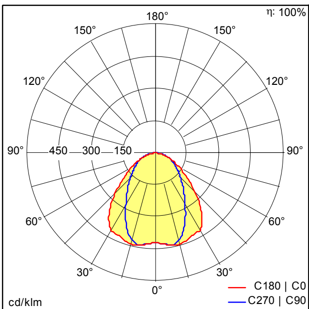
D44422AA_TEC_LED5200-865_L1000_VWB_LDE_SR_IP.ltd
