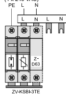
TN-S-/TT-System
