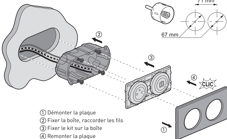
Gabarit de perçage réf. 0 905 40
