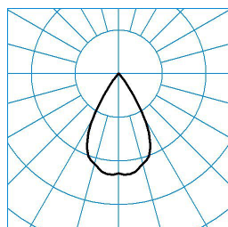
SNS ACT-CW RC3-WR1VFL-14 ■ C0 - C180
