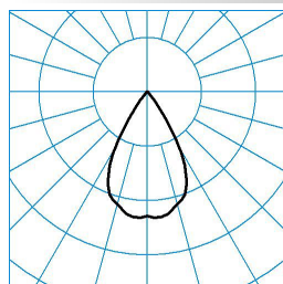
SNS ACT-WW RC3-WR1VFL-14 ■ C0 - C180
