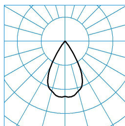
SNS ACT-SUM RC3-WR1VFL-14 ■ C0 - C180
