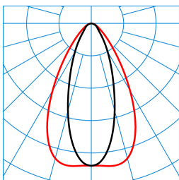
E-Line PRO 78IP50 MironaF T 270-840 ETDD L225 01 ESG Blank (LEO3) TX720043
