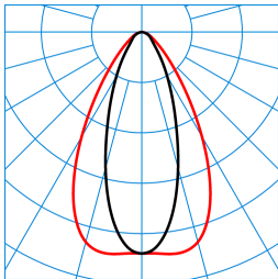
E-Line PRO 78IP50 MironaF T 270-840 ETDD L225 01 ESG Blank (LEO1) TX720014
