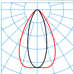
E-Line PRO 78IP50 MironaF T 270-840 ETDD L225 01 ESG 01 (LEO1) TX719921
