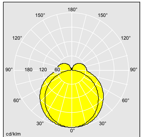
TLTP_EQUM_L1180_LED2100_840END.idt
