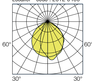
Escalier - code : 2012 0400
