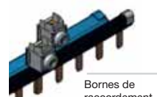
1 peigne Phase + 1 peigne Neutre
