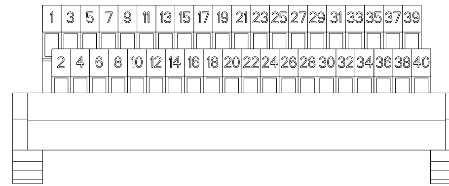
Unten / Bottom
