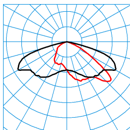
LIQ 70N-AB7L-LR-SLR2/7500-740 8G1 ET (CLO initial value) TX277755
