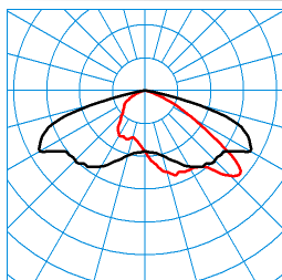
LIQ 70N-AB7L-LR-SLR2/7500-740 8G1 ET (CLO end value) TX277890
