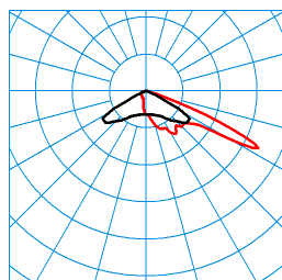
LnPlus 60-AM19L-LR/20000-722 16G1 ET (CLO initial value) TX377677 ■ C0 - C180 ■ C90 - C270 DIN 5040: A30 UTE: 1,00 J CEN Flux Code: 28 76 99 100 100
