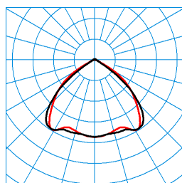
TX053207 UGR I = 20.1 UGR q = 18.9 DIN 5040: A40 UTE: 0,98 C + 0,02 T ■ C0 - C180 ■ C90 - C270
