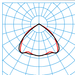
TX040383 UGR I = 21.7 UGR q = 20.7 DIN 5040: A40 UTE: 0,98 C + 0,02 T ■ C0 - C180 ■ C90 - C270
