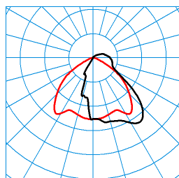
TX044683 DIN 5040: A40 UTE: 0,92 D + 0,08 T ■ C0 - C180 ■ C90 - C270
