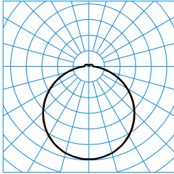
Olisq QWD2 DW 35-830 ET HFS IP54 IK + Olisq QWD2 ZDR 1/2 01 TX461136
