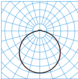
Olisq QWD2 DW 35-830 ET HFS IP54 IK + Olisq QWD2 ZDR 1/2 03 TX460761
