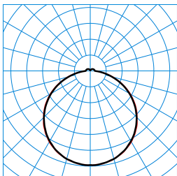
Olisq QWD2 DW 35-830 ET HFS IP54 IK + Olisq QWD2 ZDR 1/2 05 TX461565
