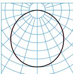
Olisq QWD2 DW 35-830 ET HFS IP54 IK + Olisq QWD2 ZDR 1/1 01 TX461736
