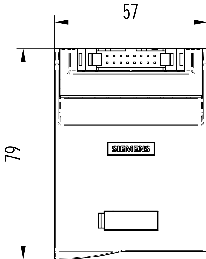
Vorne / Front
