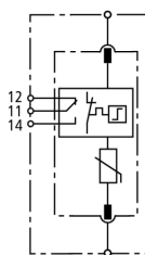
Schéma de principe du circuit DG S 600 FM
