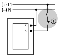
① Arrêt d'urgence (coupure d'urgence)
