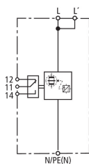
Schéma de principe du circuit DBM 1 760 FM
