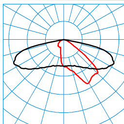
LIQ 50N-AB2L-LR-SLR2/6800-740 6G1 ET (CLO end value) TX278158
