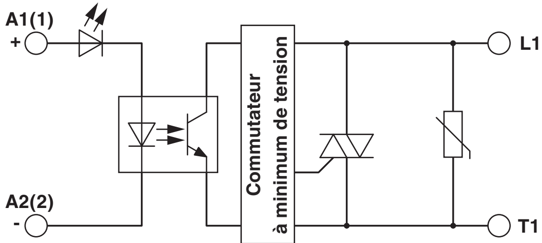
Schéma fonctionnel
