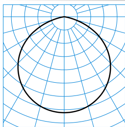
Combial 45 G2 RB8L/150-250/3/ML-MC G1 ET (stage 1) ■ C0 - C180 TX711697
