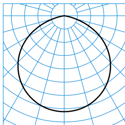
Combial 45 G2 RB8L/150-250/3/ML-MC G1 ET (stage 2) ■ C0 - C180 TX711702
