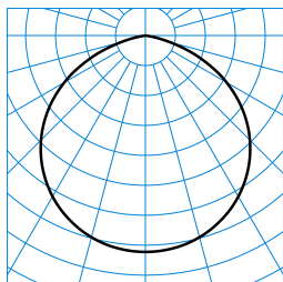
Combial 45 G2 RB8L/150-250/3/ML-MC G1 ET (stage 3) ■ C0 - C180 TX711711
