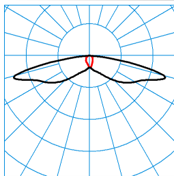
Jovie 50-SB3L-LRA/1000-740 2G1 ET TX068587 ■ C0 - C180 ■ C90 - C270 DIN 5040: A20 UTE: 1,00 l CEN Flux Code: 29 61 91 100 100
