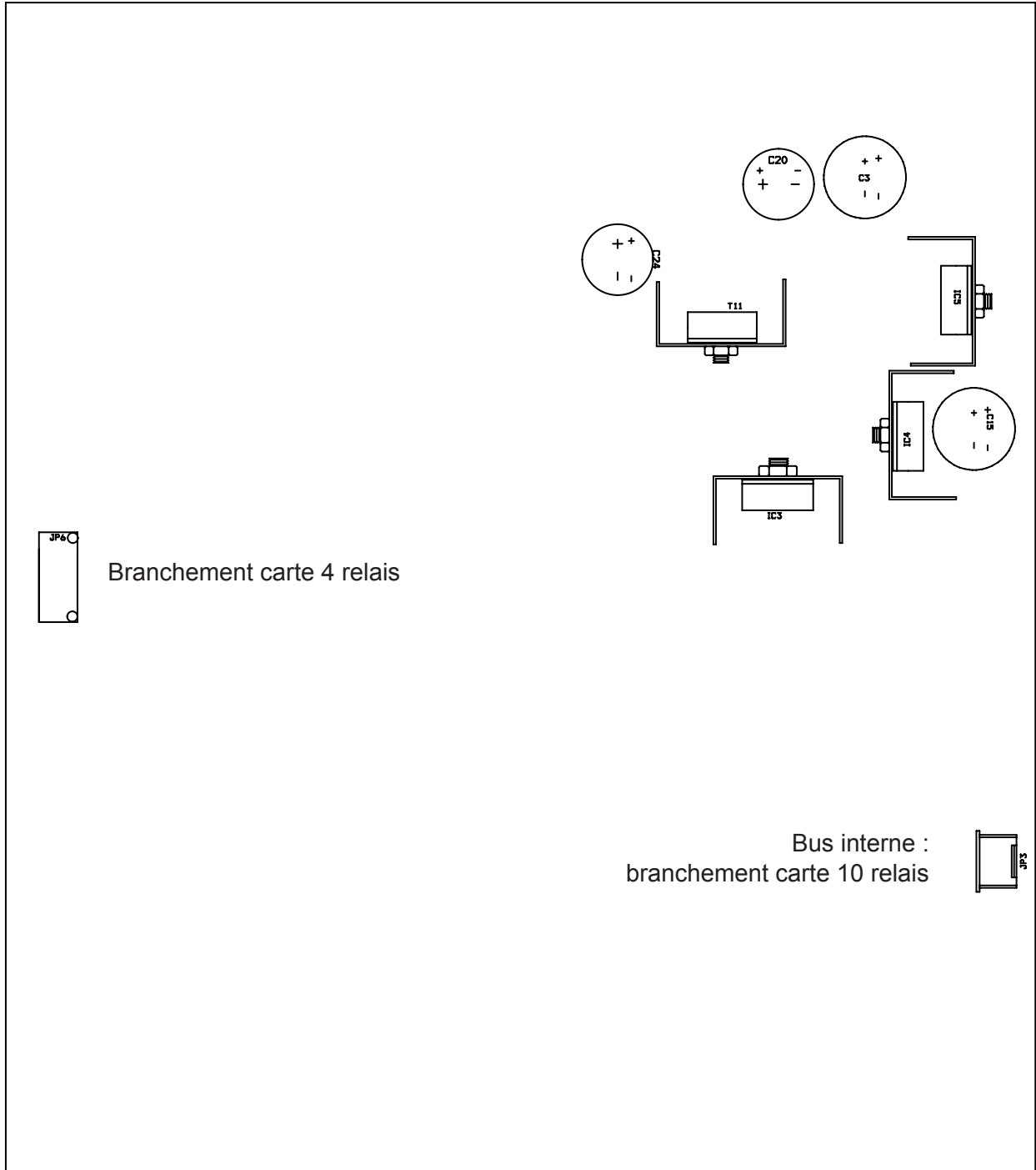
Carte électronique principale vue de dessous (boîtier ouvert)
