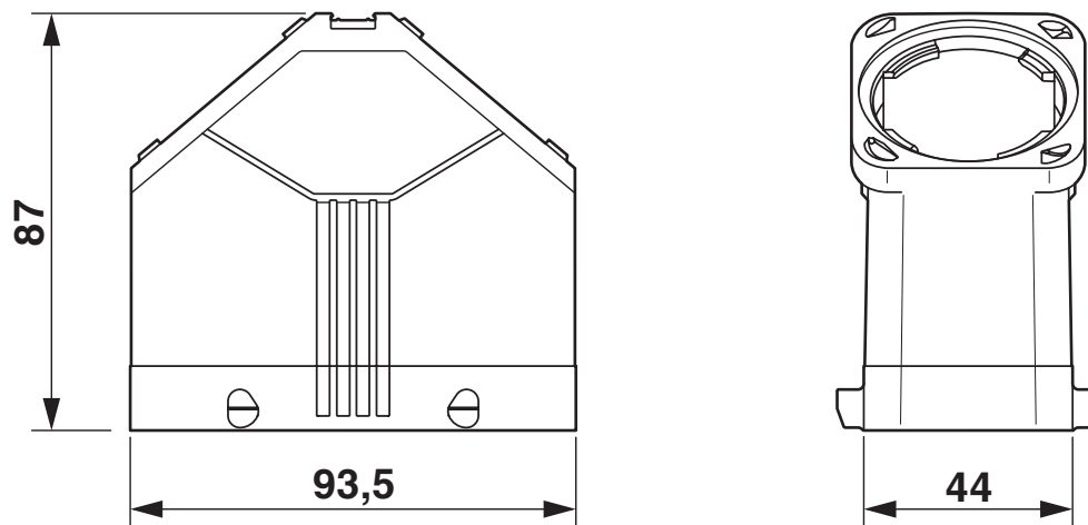
Dessin coté
