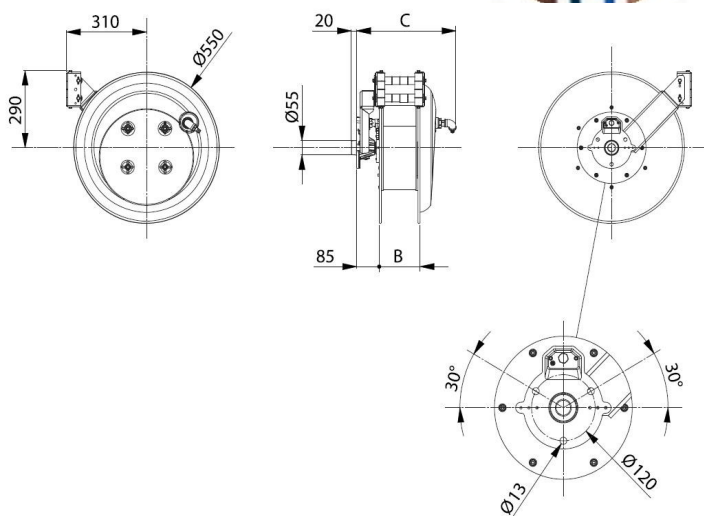
Dimension sans bride
