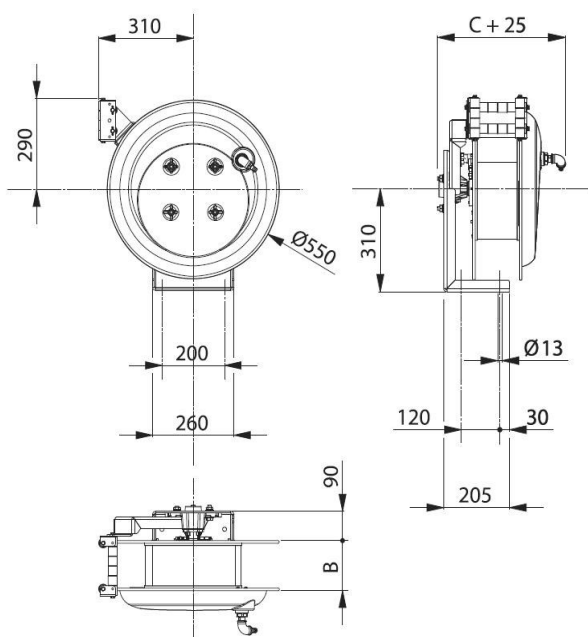
Dimension avec bride
