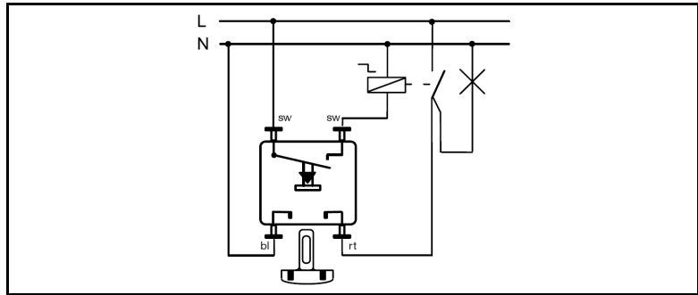
Schémas de raccordement 534 U
