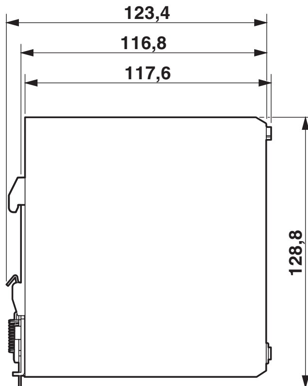
Dessin coté
