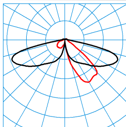
8841LS-Ü 260-AB2L/2400-730 3G2 ET (CLOANFANGSWERT) TX369253 C0 - C180 C90 - C270 DIN 5040: A20 UTE: 0,92 I + 0,08 T CEN Flux Code: 28 63 91 92 100 13 34 62 8
