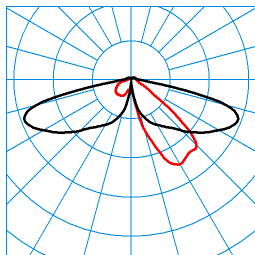
8841LS-Ü 260-AB2L/2400-730 3G2 ET (CLOENDWERT) TX369422 C0 - C180 C90 - C270 DIN 5040: A20 UTE: 0,92 I + 0,08 T CEN Flux Code: 28 63 91 92 100 13 34 62 8
